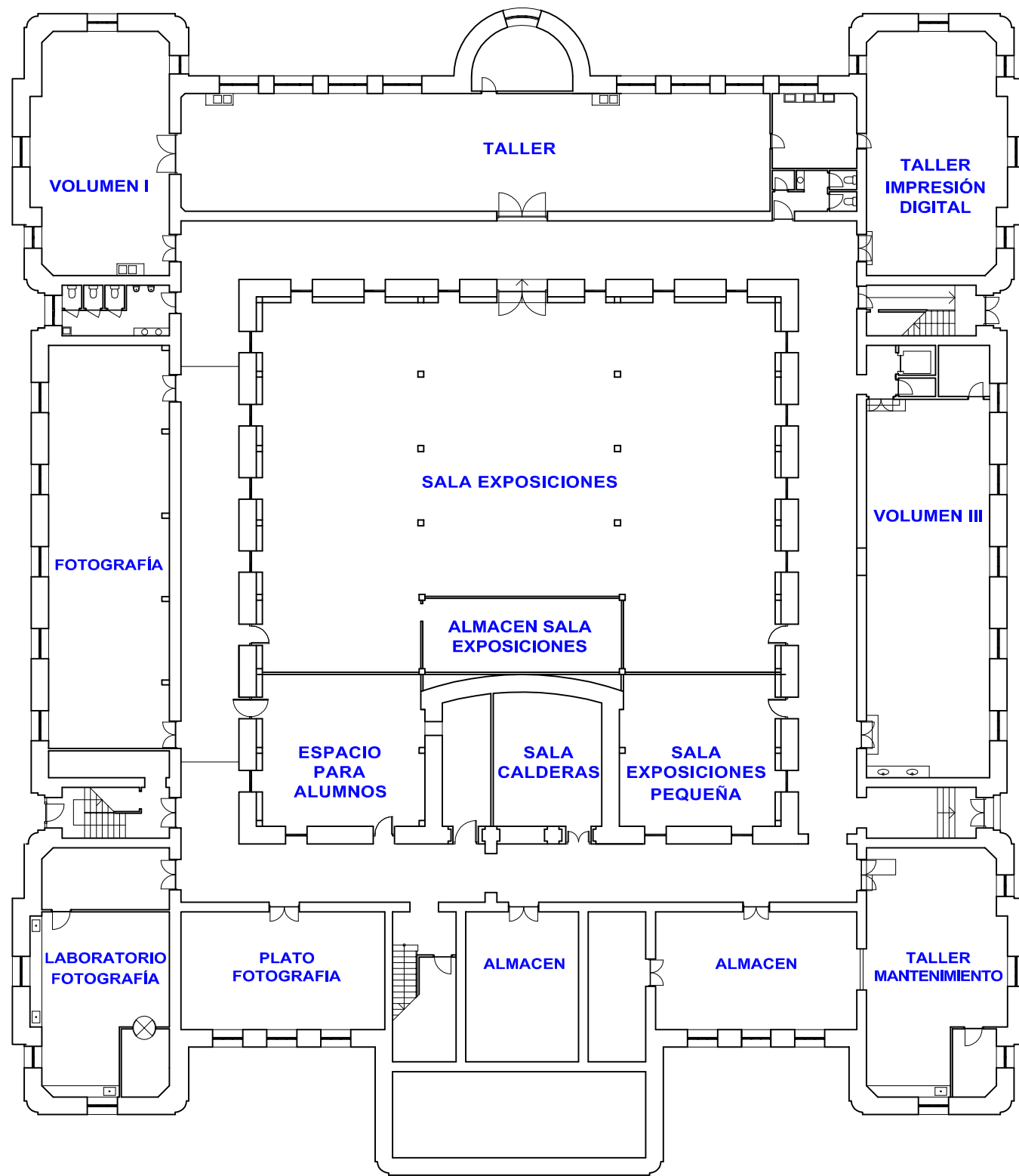
PLANTA SOTANO
