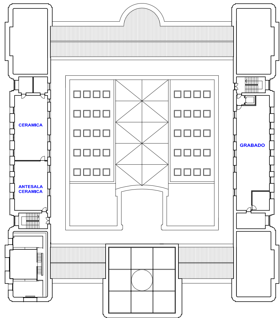
PLANTA SEGUNDA
